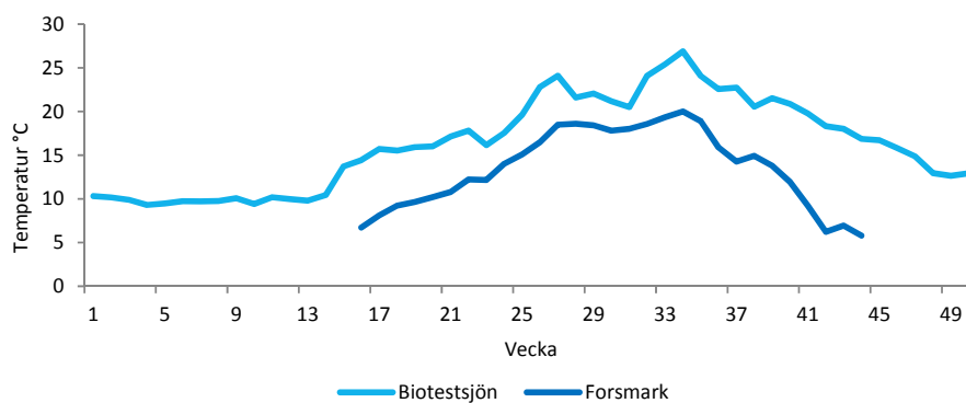
Figur 2. Medeltemperaturer per vecka i Biotestsjön (centralt i Biotestsjön) och Forsmark (Ön) under år 2015.
