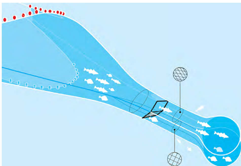
Art separerande rist i trål med två lyft. Plattfisk fångas i undre lyftet och stor rundfisk i övre lyftet.
